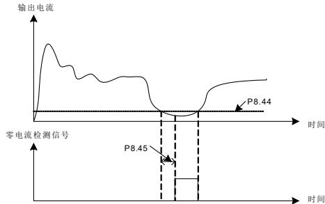
图 6-22 零电流检测示意图
