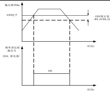
图 6-19 FDT 电平示意图
