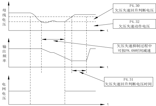
欠压失速抑制示意图
