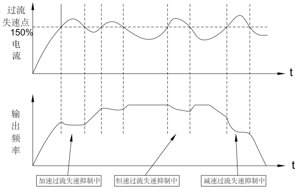
图 6-10-1 VF 过流抑制示意图
