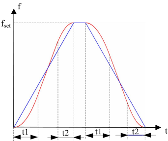
图 6-16 S 曲线加减速 A 示意图
