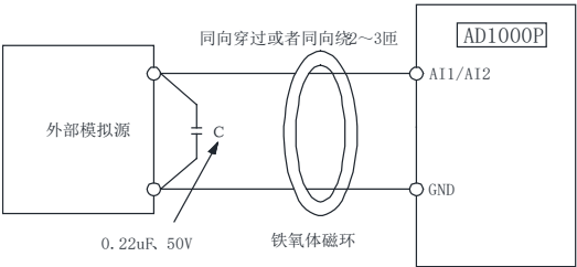
图 3-3 模拟输入端子加滤波处理接线图
