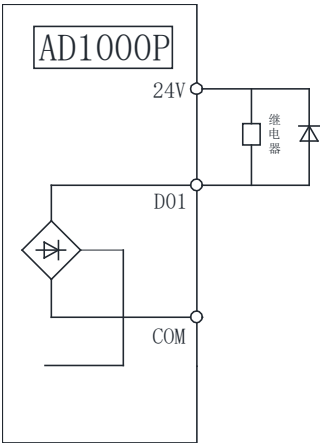
图 3-6 使用内部电源驱动外部继电器接法
