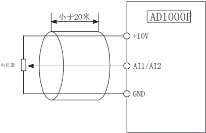
图 3-2 模拟输入输出端子接线示意图
