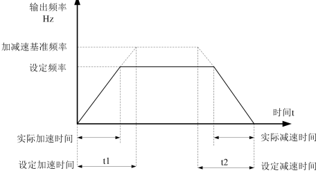
图 6-1 加减速时间示意图
