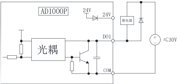
图 3-7 使用外部电源驱动继电器接法
