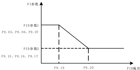
图 6-26 PID 参数切换
