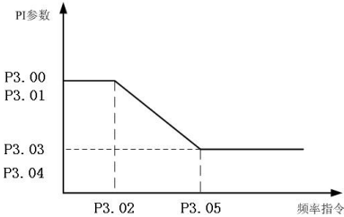
图 6-8 PI 参数示意图
