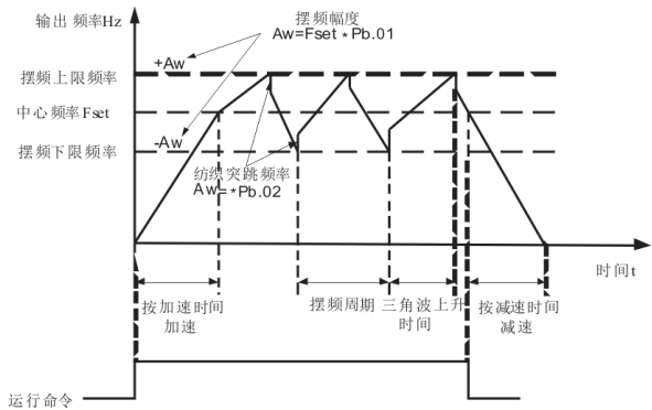
图 6-28 摆频工作示意图
