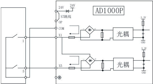
图 3-4 使用内部电源干接点方式，S7 端子 H 位短接
