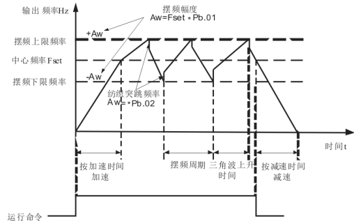
图 6-28 摆频工作示意图
