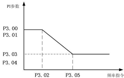
图 6-8 PI 参数示意图
