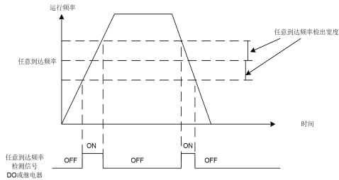
图 6-21 任意到达频率检测示意图
