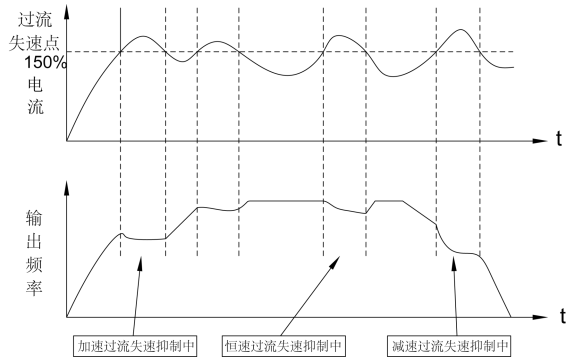
图 6-10-1 VF 过流抑制示意图
