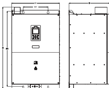
图四(扁平尺寸图)
