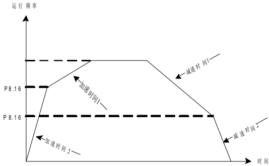
图 6-15 加减速时间切换示意图
