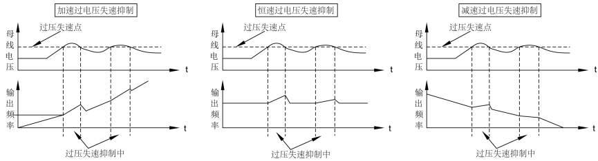
过压失速动作示意图
