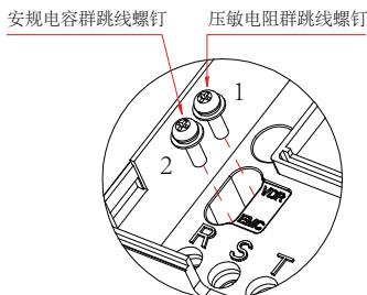
压敏电阻 (VDR)、安规电容 (EMC) 对地跳线位置示意图
