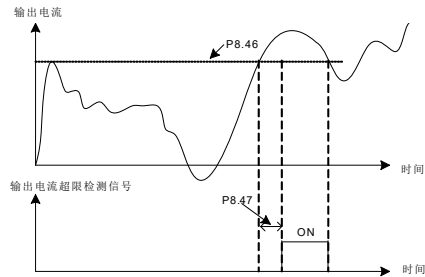
图 6-23 软件过流点示意图
