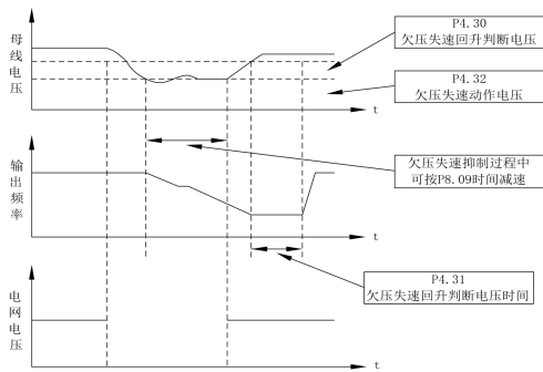
欠压失速抑制示意图
