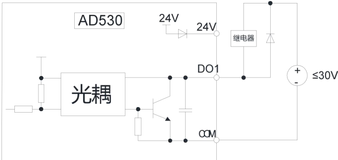
图 3-7 使用外部电源驱动继电器接法
