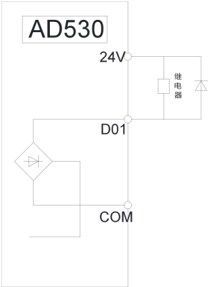
图 3-6 使用内部电源驱动外部继电器接法
