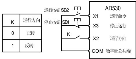
图 6-6 三线式模 2
