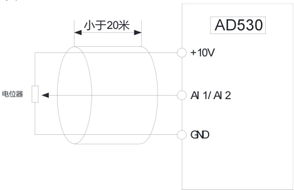
图 3-2 模拟输入输出端子接线示意图
