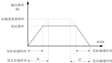
图 6-1 加速时间示意图
