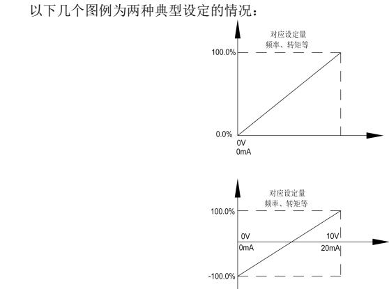
图 6-11 模拟给定与设定量的对应关系
