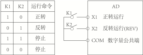
图 6-2 两线式模式 1
