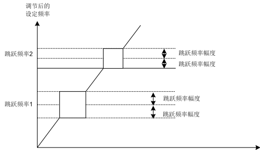
图 6-13 跳跃频率示意图
