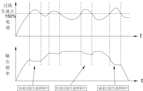
图 6-10-1 VF 过流抑制示意图
