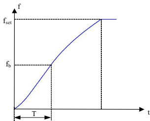
图 6-17 S 曲线加减速 B 示意图
