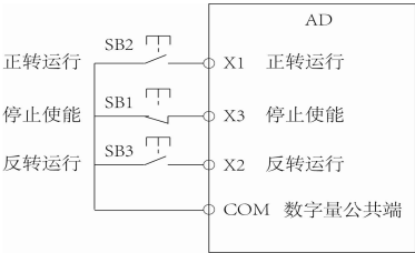
图 6-4 三线式模式 1（常闭启动）
