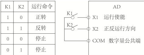
图 6-3 两线式模式 2
