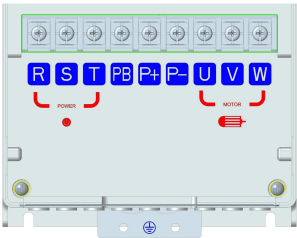
（正面图）
